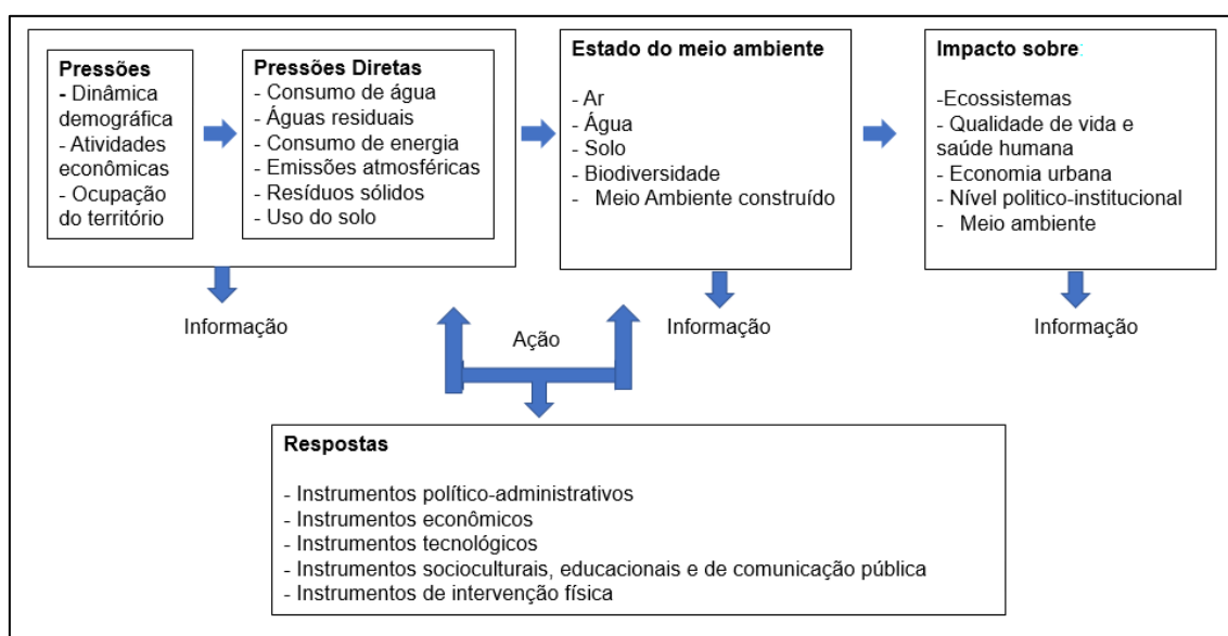
Figura 1 – Matriz PEIR e as interações dos componentes urbano-ambientais
